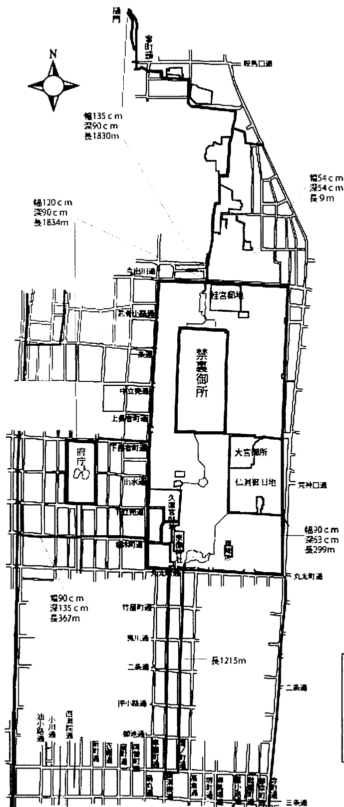
図-2 明治23年着工の疏水分線からの御所用水及び御苑外用水の水路地図(京都府立総合資料館文書 文献20を筆者がトレースし、水路幅・深さ・長さを加筆した)
