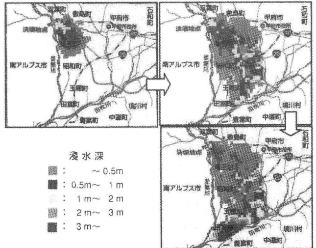
図-3 釜無川の信玄堤付近が決壊した場合の浸水被害想定シミュレーション 9)
