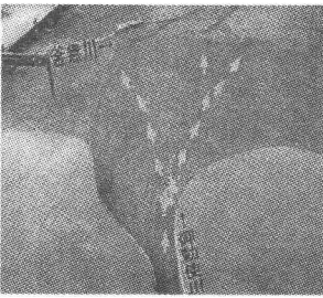
図-22 土砂供給を15cc/分とした時の流路形成
