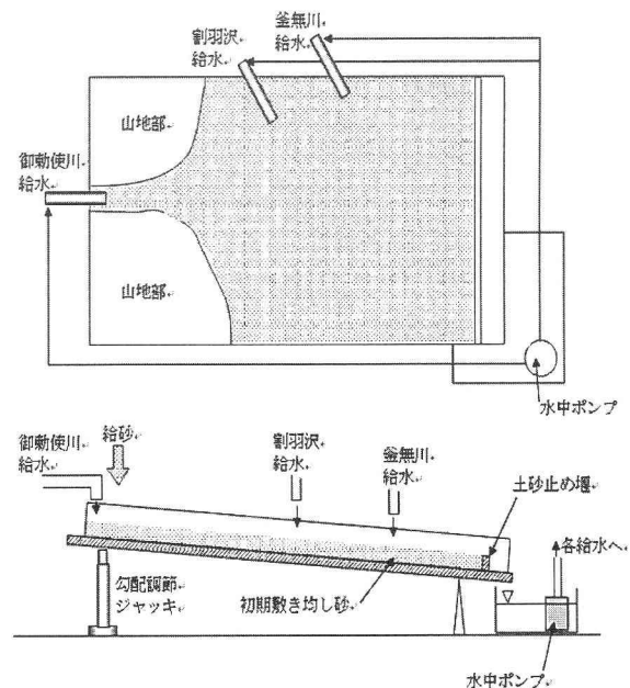
図-17 御勂使川扇状地モデル縦横断面図
