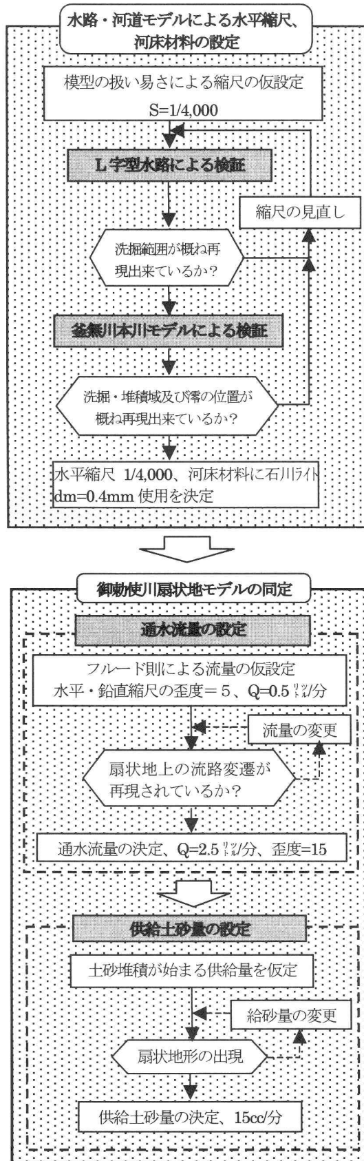
図-18 実験条件設定のフロー図
