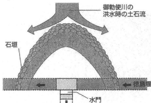
図-13 徳島堰の小将棋頭のイメージ平面図
