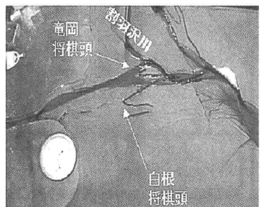
図-29 2つの将棋頭による流れ
