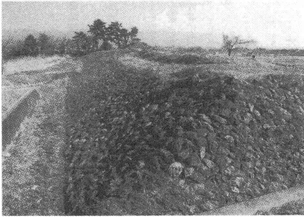
写真-3 白根将棋頭
