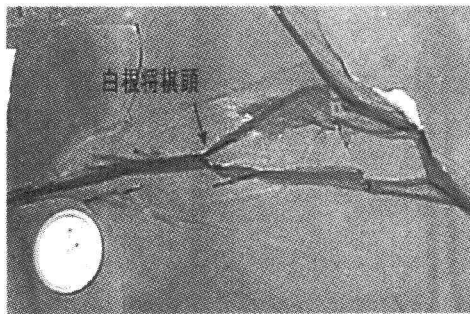
図-26 供給土砂量1倍時に将棋頭で二分した流路
