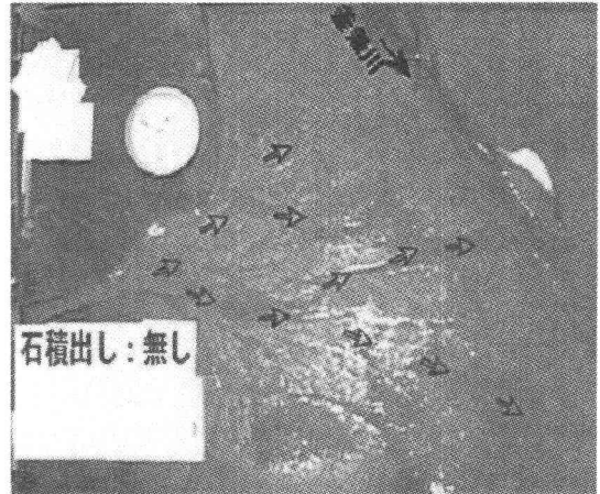
図-24 石積み出しを設置しない場合の流路の変遷状況
