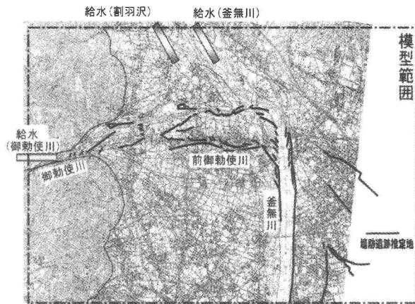
図-16 御勂使川扇状地モデルの対象範囲
