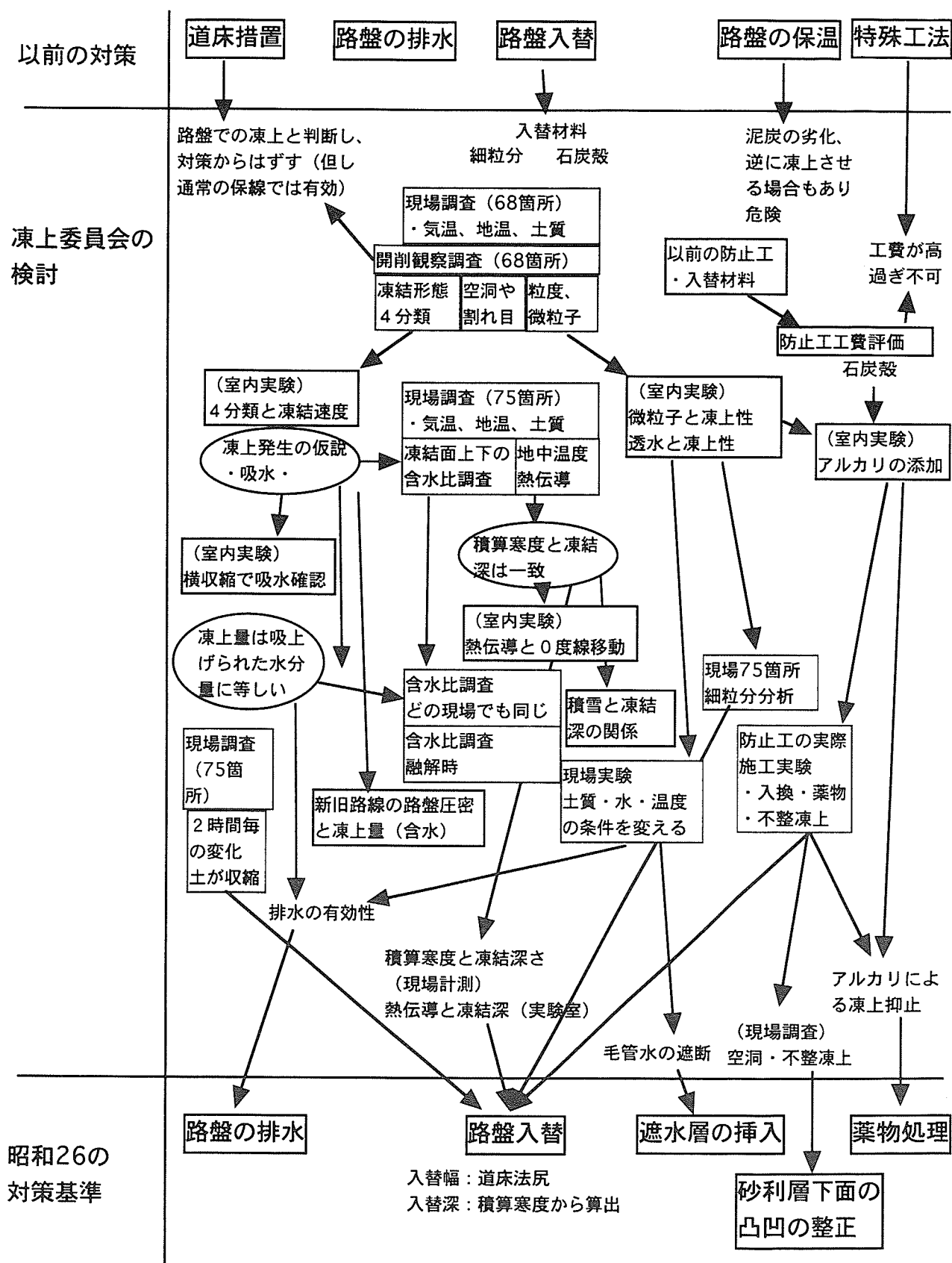
図9 凍上対策研究委員会における研究と対策工の変遷（原口作成）
