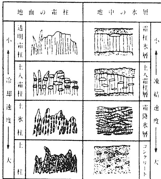
図7 霜柱と凍上の類似 注6
