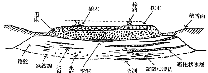
図9 中谷宇吉郎が観察した線路凍上の被害状況 注8
