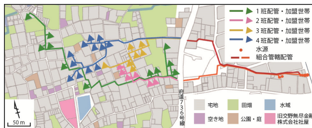
図-5 1983（昭和58）年時点での倉治取水組合配管図 『水源井戸及び配管位置図』をもとに筆者作成
