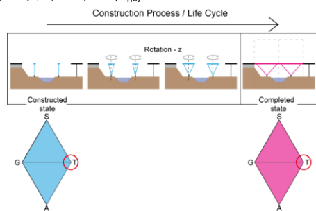
図-20 構造形態の推移 (キングスゲート橋)
