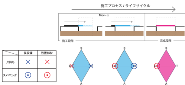
図-10 施工プロセス/ライフサイクルダイアグラムの例（送出し工法）
