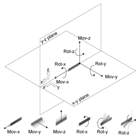
図-8 橋梁の移動・回転の定義
