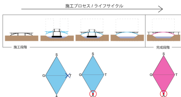
図-16 構造形態の推移 (ピース橋)
