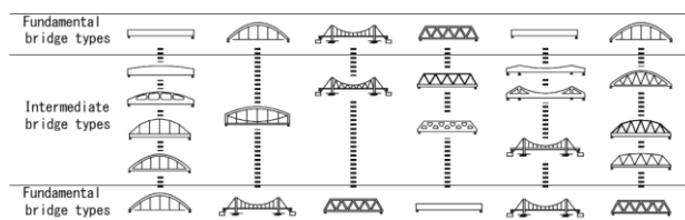
図一5 基本橋梁形式間の連続的關係性 [久保田 2010]
