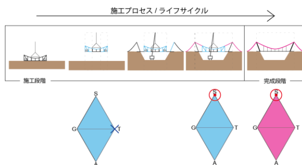
図-14 構造形態の推移（ハルゲイバー橋）
