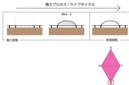
図-18 構造形態の推移 (多摩大橋)
