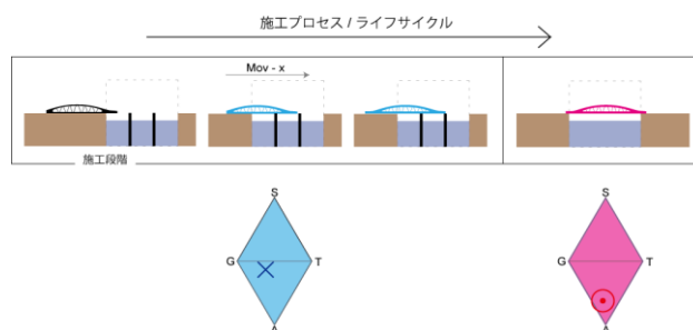
図-22 構造形態の推移 (新豊橋)
