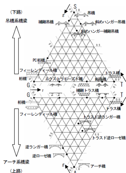
図一6 三角座標表示による構造形態相関図 [久保田 2010]
