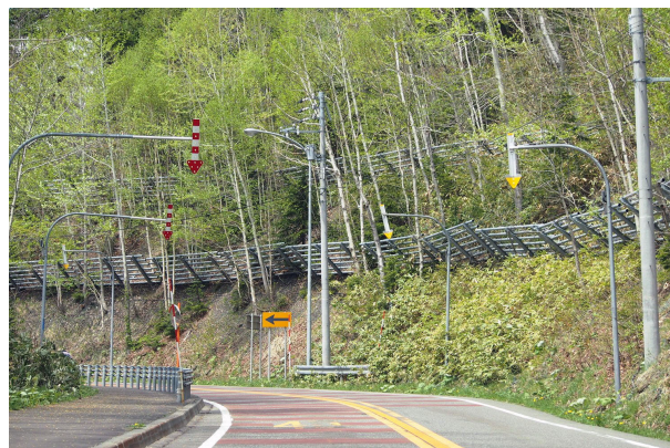
写真-1 北海道の道路に設置された多数の道路付属物
