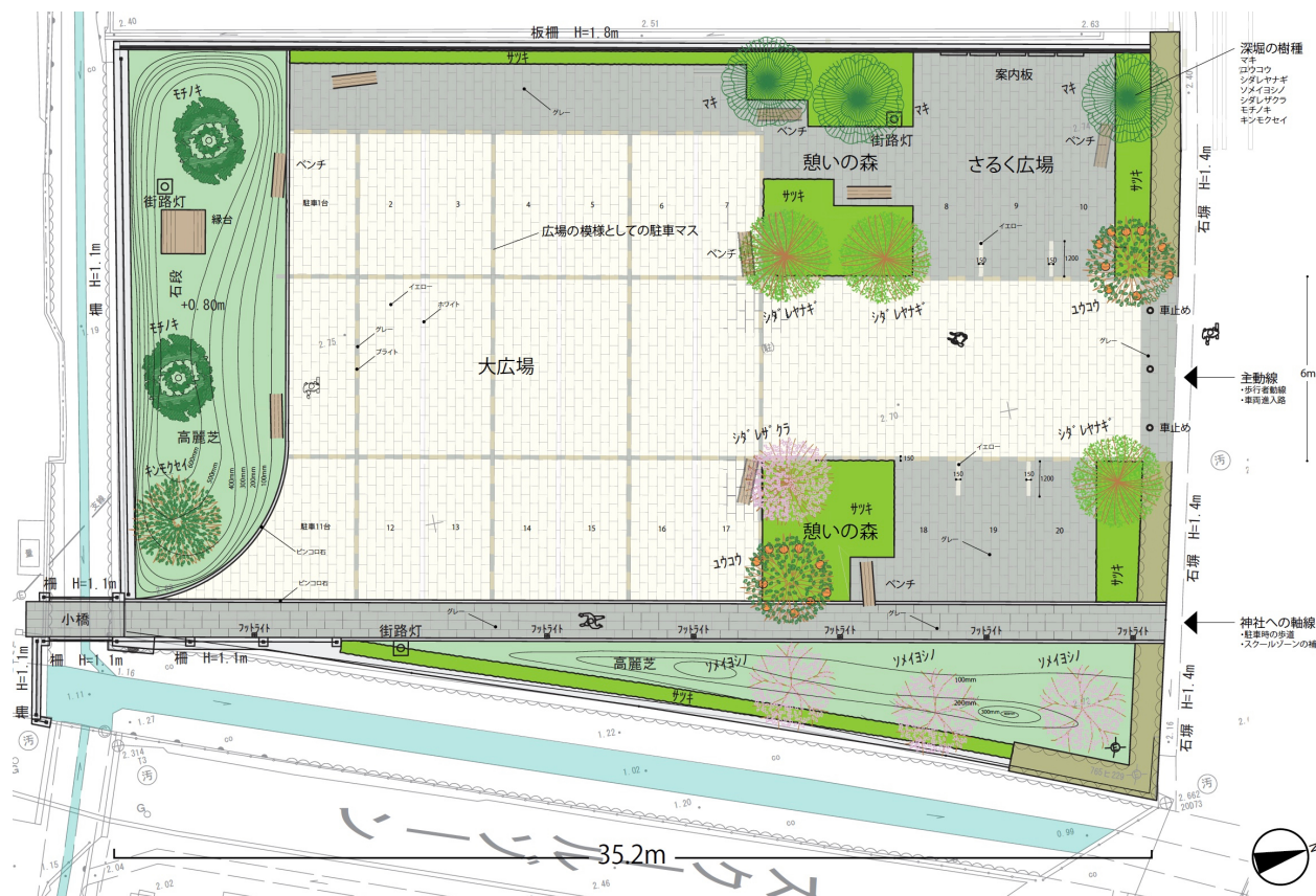
図-6 配置計画（最終）
