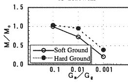
(d) Reduction Ratio of Bending Moment of Center Wall
