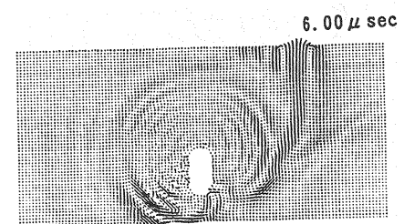
(d) Angled wave method ; slot hole
