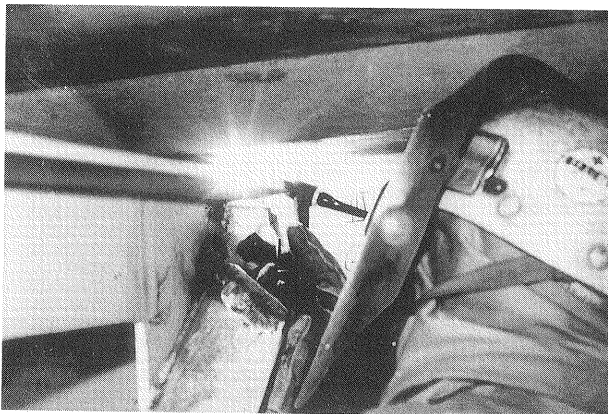
Photo2 Repairing of actual bridge.
