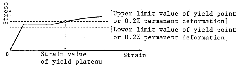
Fig. 1—Strain value of yield plateau.
