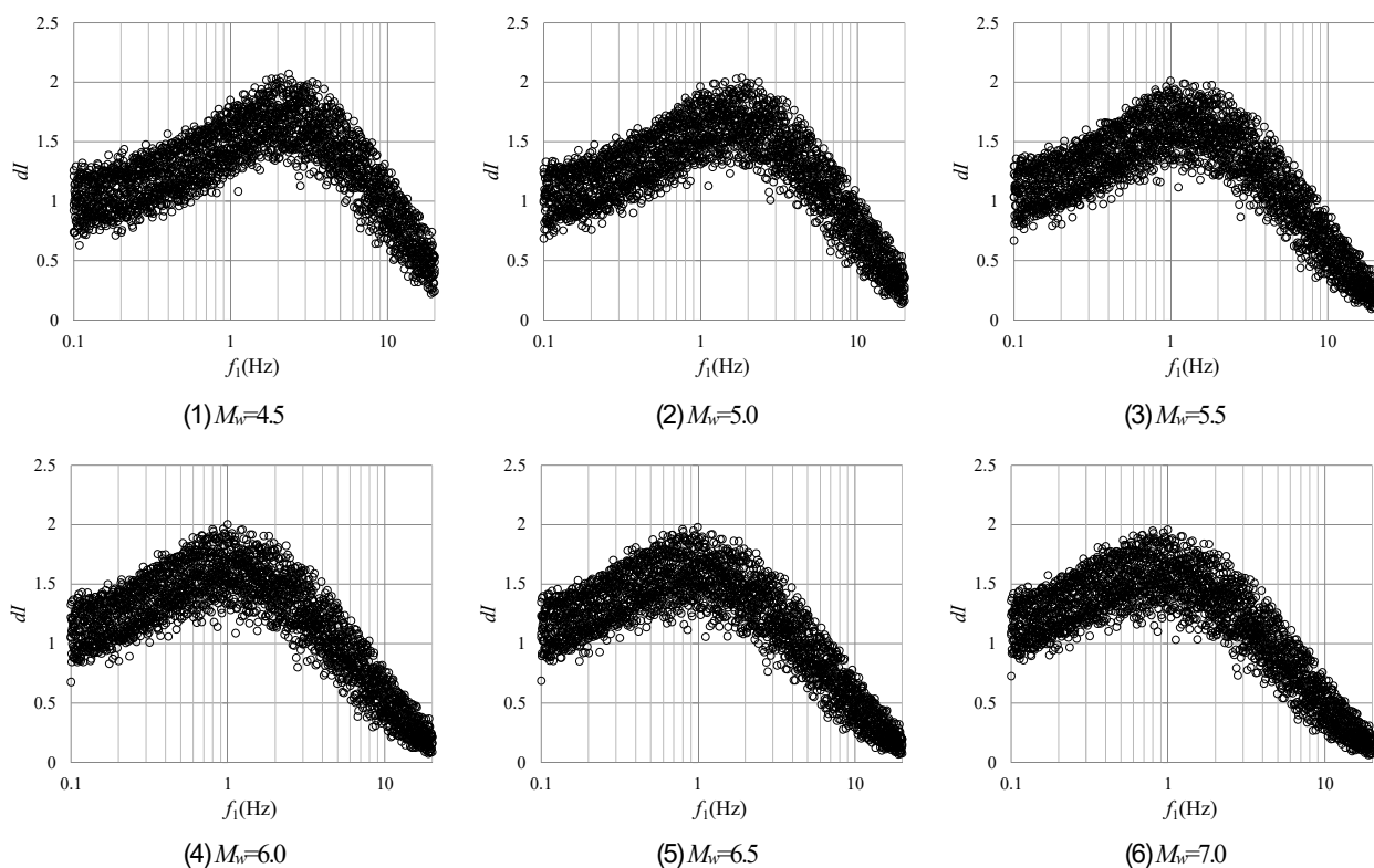
図-5 1次ピーク振動数 f_1 と式(8)による震度増分 dI の対応 (プレート境界地震, f_{max}=6\text{Hz} )
