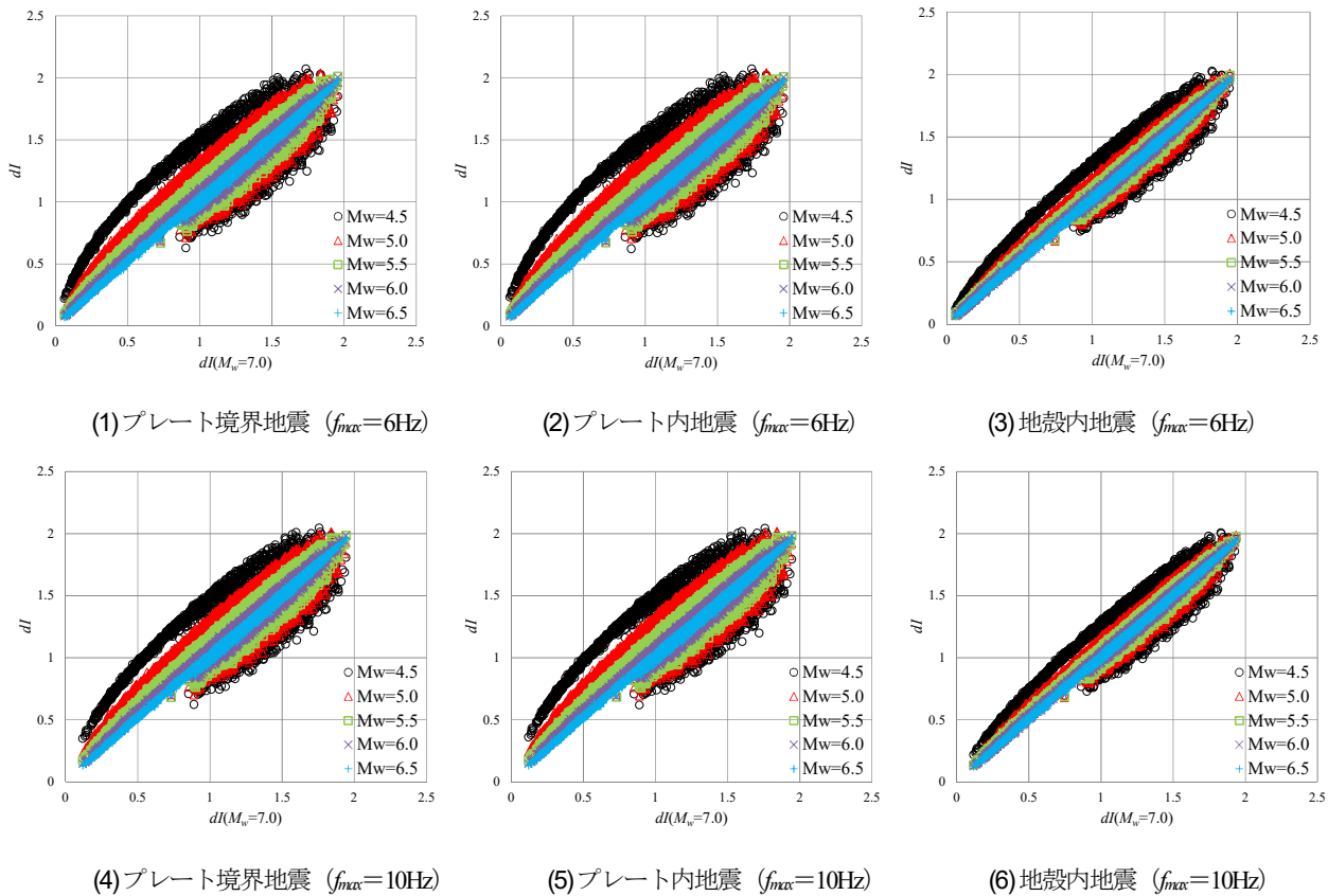
図-11 M_w=7 の震度増分 dl と M_w=4.5\sim 6.5 の震度増分 dl の対応
