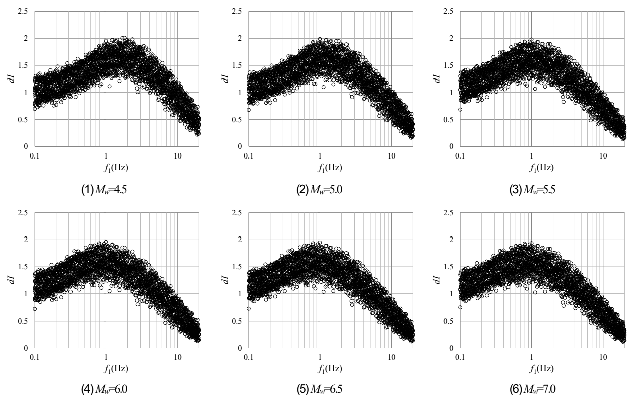
図-10 1次ピーク振動数 f_1 と式(8)による震度増分 dI の対応（地殻内地震， f_{max}=10\text{Hz} ）
