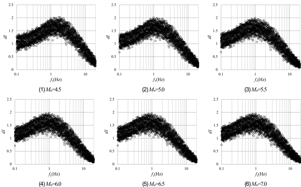
図-9 1次ピーク振動数 f_1 と式(8)による震度増分 dI の対応（地殻内地震， f_{max}=6\text{Hz} ）
