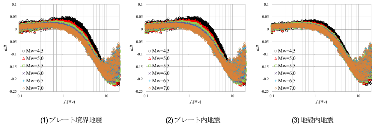
図-12 f_1 と dI の対応
