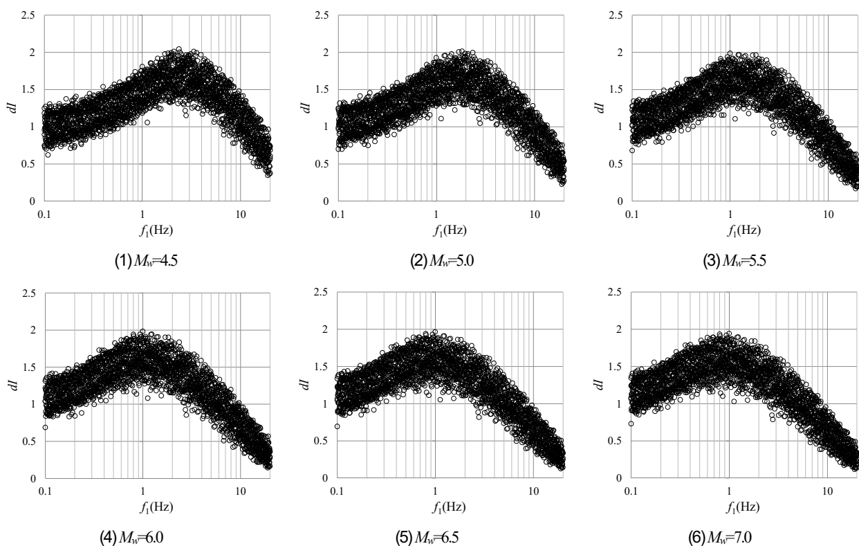
図-6 1次ピーク振動数 f_1 と式(8)による震度増分 dI の対応 (プレート境界地震, f_{max}=10\text{Hz} )
