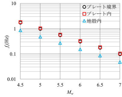
図-4 M_w とコーナー振動数 f_c
