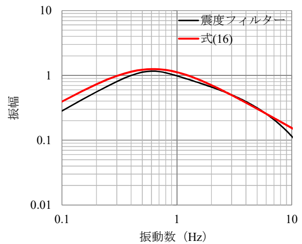
図-1 震度フィルターと式(16)の対応
