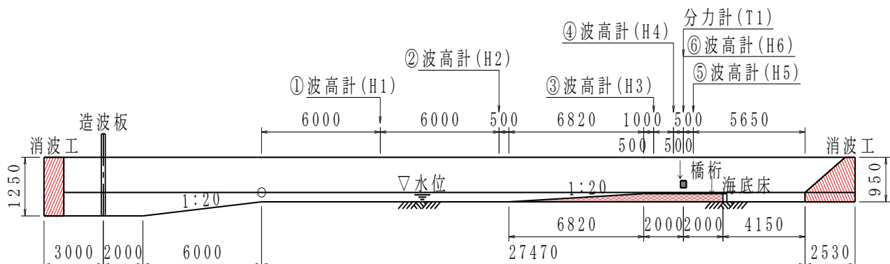
図－1 実験水路
