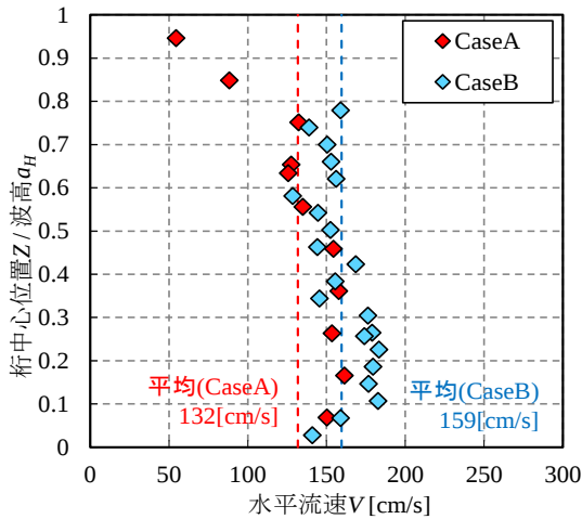
図-1 3 流速分布
