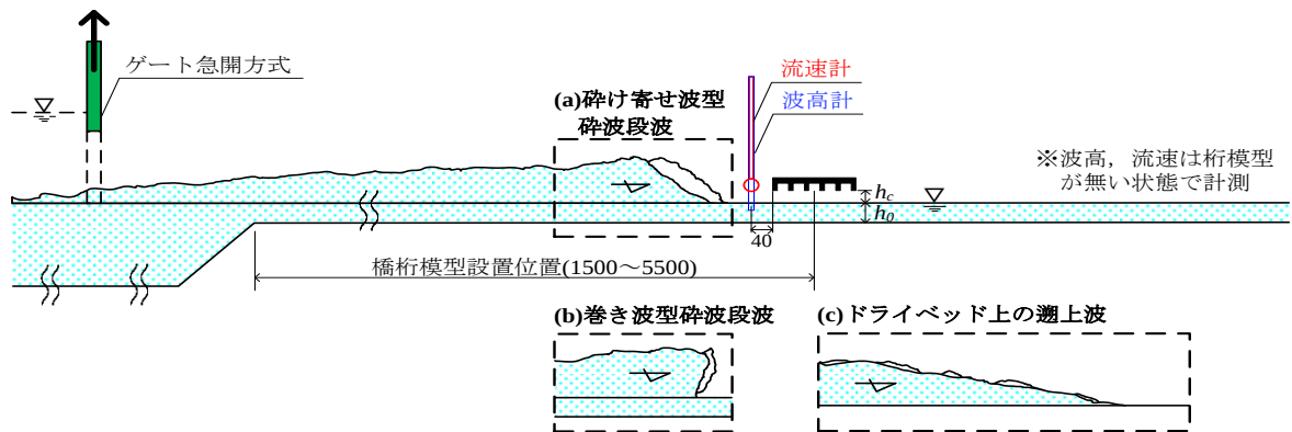
図－４ 庄司らの実験波形状
