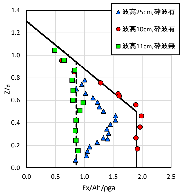
図-3 桁下高、波高をパラメータとした実験結果
