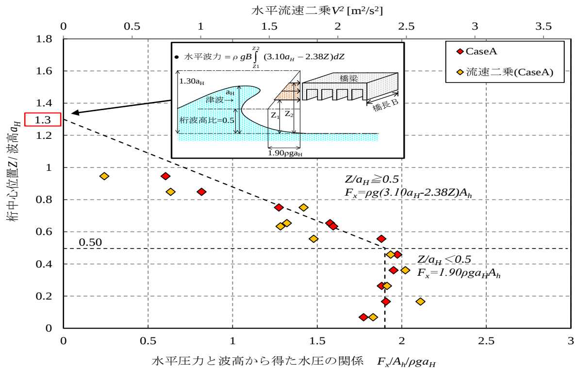
図-11 F_x/A_h/\rho g a_H と V^2 の関係
