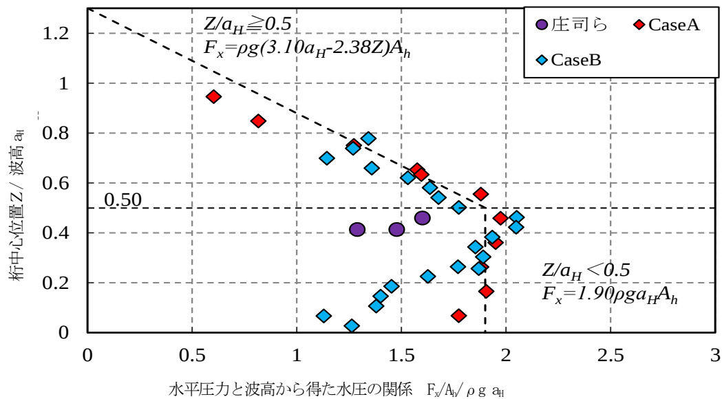
図-1 4 桁位置と水平波圧（補正後）
