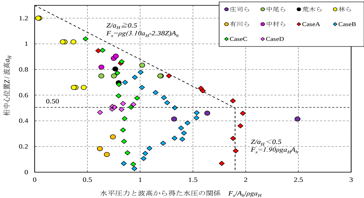
図-10 桁位置と水平圧力/波高から得られた水圧の関係
