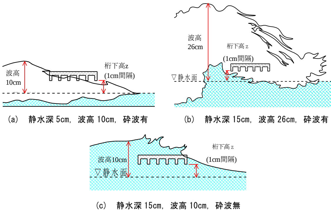
図-2 実験状況模式図と実験パラメータ
