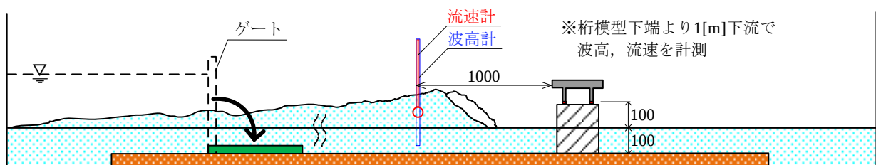
図－５ 中尾らの実験波形状
