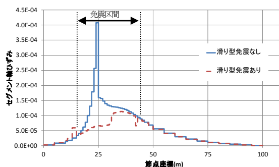
図-2 滑り型免震構造の有無とセグメント軸ひずみ
