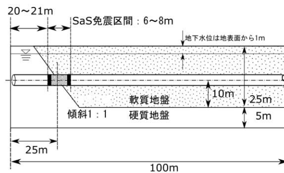
図-6 SaS 免震の適用範囲と地盤条件
