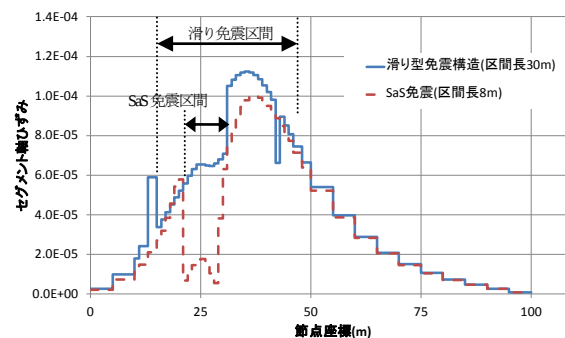
図-8 滑り型免震構造と局所的に配置した SaS 免震の比較
