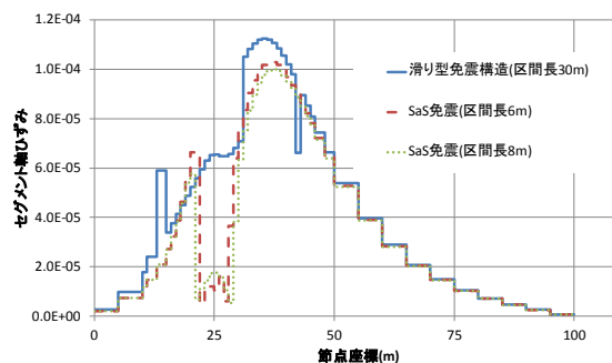
図-7 滑り型免震構造と SaS 免震の比較
