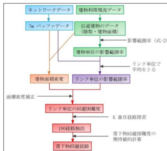
図-2 避難経路抽出のフロー
