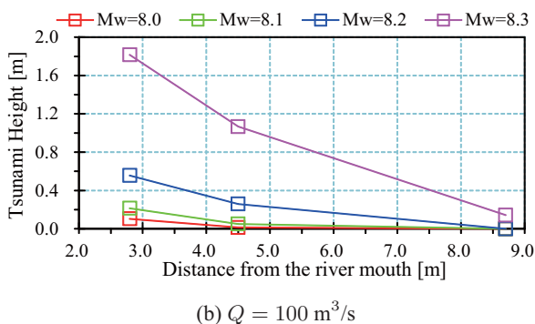
図-5 流量別の各施設地点における第1波の波高
