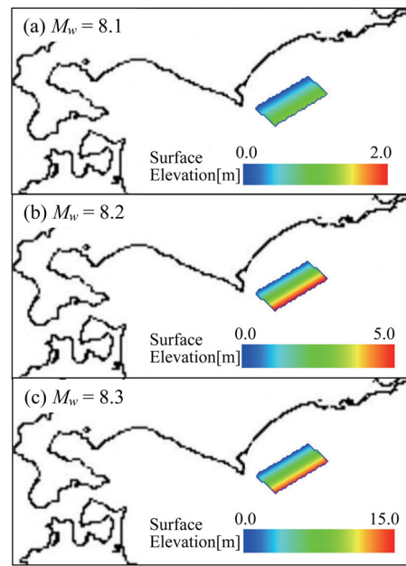
図-3 各 M_w に対する十勝沖地震津波の初期水位分布
