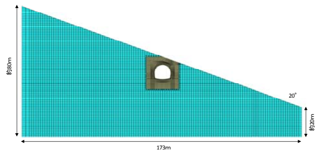
(a) 解析メッシュ (斜面角 20 度)
