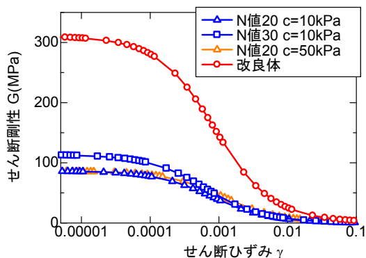
(a) せん断剛性-せん断ひずみ関係
