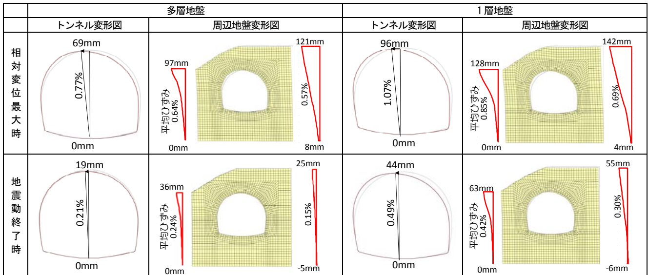
図-7 トンネルおよびトンネル周辺地盤の変形図
