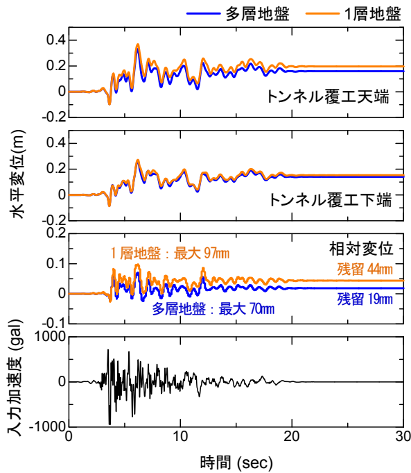
図-8 トンネル覆工の変位時刻歴
