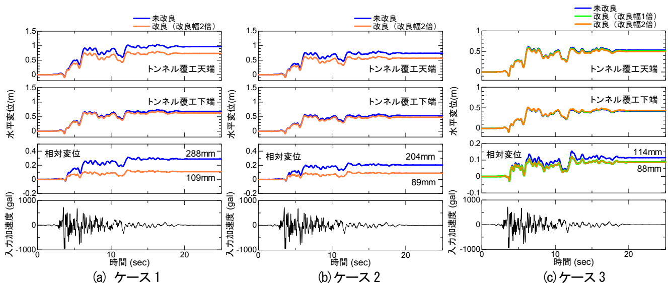
図-12 改良効果の検討：トンネル覆工の水平変位時刻歴
