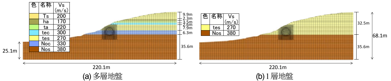
図-6 検討に用いた斜面
