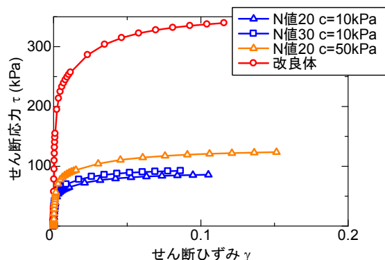
(b) せん断応力-せん断ひずみ関係
