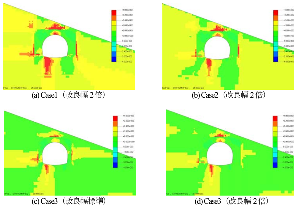
図-13 改良効果の検討：残留せん断ひずみ分布
