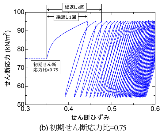
図-5 初期せん断を与えた繰返し中空ねじり試験結果の例
