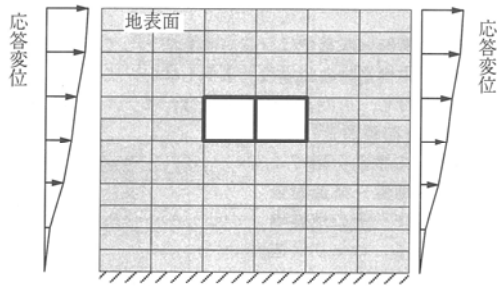
図-1 FEM 応答変位法 10)
