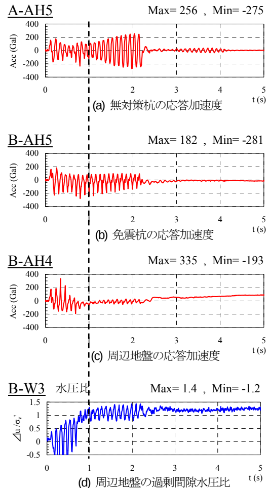
図-5 応答加速度と過剰間隙水圧比の比較
