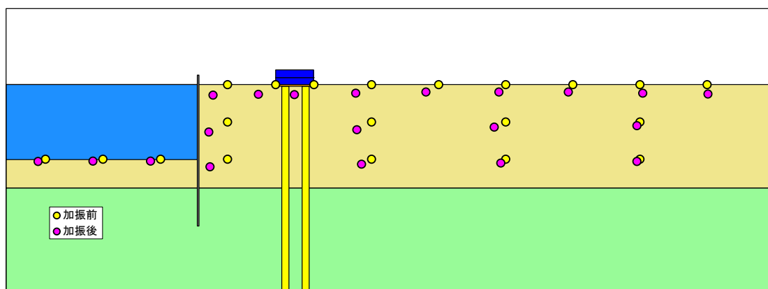
図-8 地盤の残留変位 (変形倍率: 2倍)
