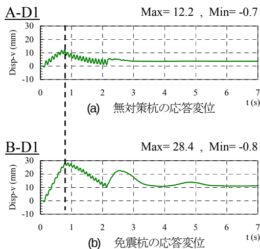
図-6 杭頭部の応答変位
