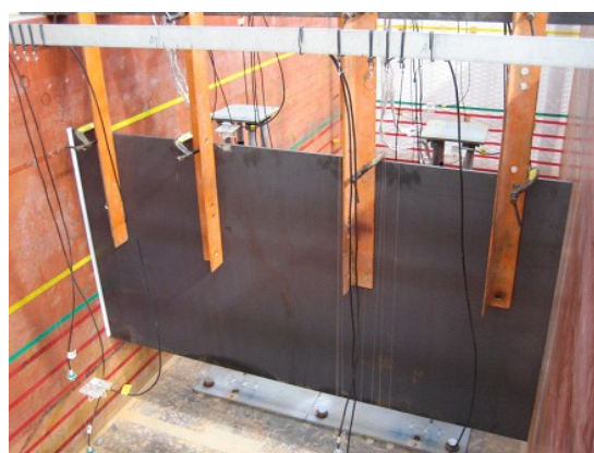
(b) 鋼板設置（治具固定）完了
