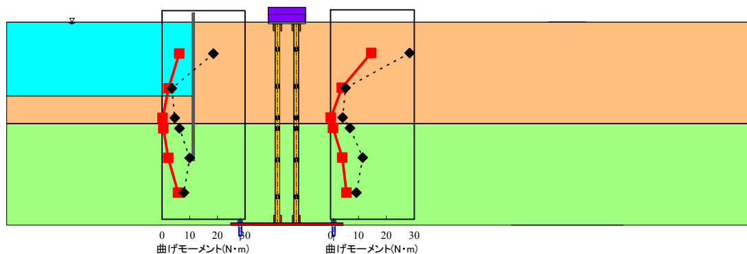
図-7 杭基礎の最大曲げモーメント分布（無対策杭と免震杭との比較）
