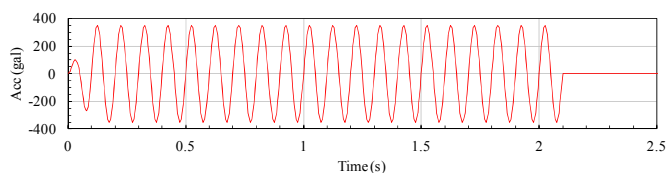
図-3 加振波 (最大加速度 350Gal)
