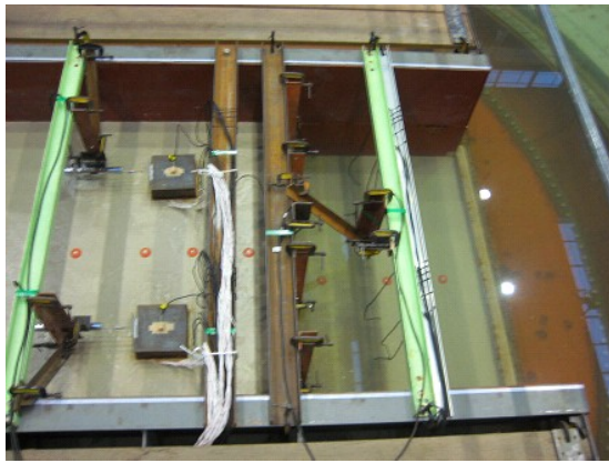
(d) 模型地盤作製完了 (前面側)
