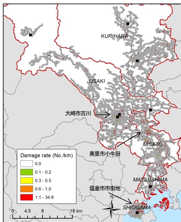
図-4 管路属性補正後の管路被害率分布 (■印は観測点)
