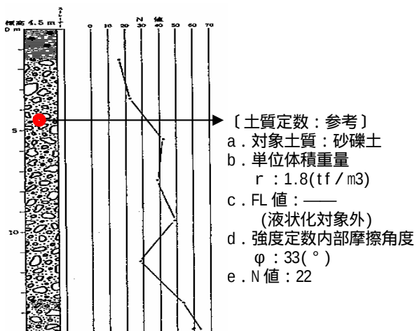
図-8 安倍川側堤防土質資料
