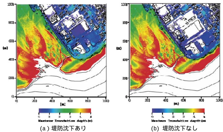
図-16 最大浸水深分布（想定東海モデル初期水位×2.0倍，）
