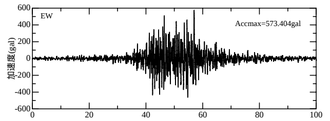
図-3 解析対象地震動 - 野津波 S2 (EW) -
