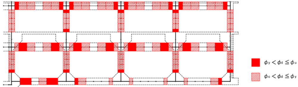
図-6 反応タンクの損傷状況
