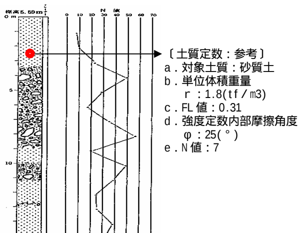
図-7 駿河湾側堤防土質資料
