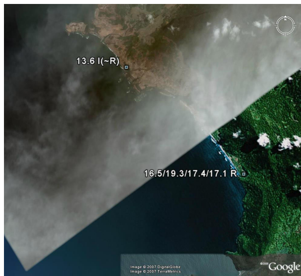
図-5 津波痕跡高(5° 7' Nから5° 13' N)
