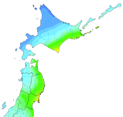
(c) 別途評価された宮城県沖・三陸沖北部地震の短周期レベルを使用
