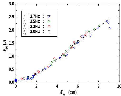
図-15 振動エネルギー E_{EQ} と水平方向の平均変位 \delta_{rs} の関係
