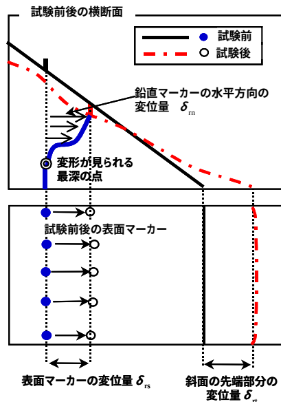
図-6 斜面水平方向の平均変位 \Delta\delta_s の評価方法
