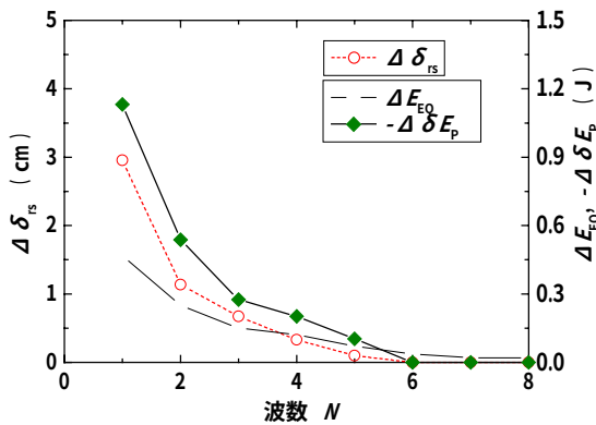
図-8 1波毎の水平方向の変位量 \Delta \delta_{rs} と振動エネルギー \Delta E_{EQ} と位置エネルギー \Delta E_p の関係 \delta_{rs} の関係
