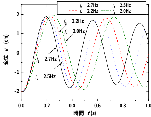
図-11 異なる振動数 f の減衰振動波形の比較
