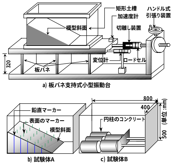
図-2 試験装置
