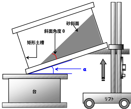
図-18 安息角の測定方法
