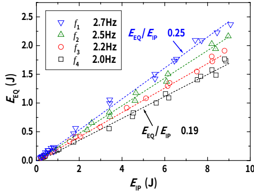
図-14 振動エネルギー E_{EQ} と入力エネルギー E_{IP} の関係
