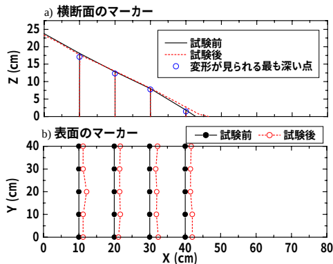
図-19 静的な試験の試験前後のマーカの動き
