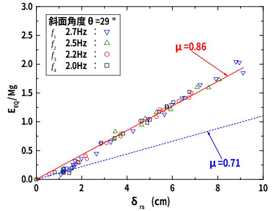
図-21 異なる振動数 f 、斜面角度 \theta の模型実験により E_{EQ}/Mg と水平方向の変位量 \delta_{rs} の関係
