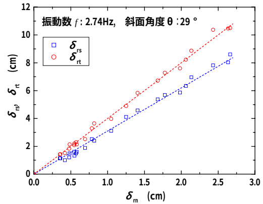
図-7 水平方向の変位量 \delta_m と斜面表面マーカーの変位量 \delta_s , 斜面先端部分の変位量 \delta_n の関係
