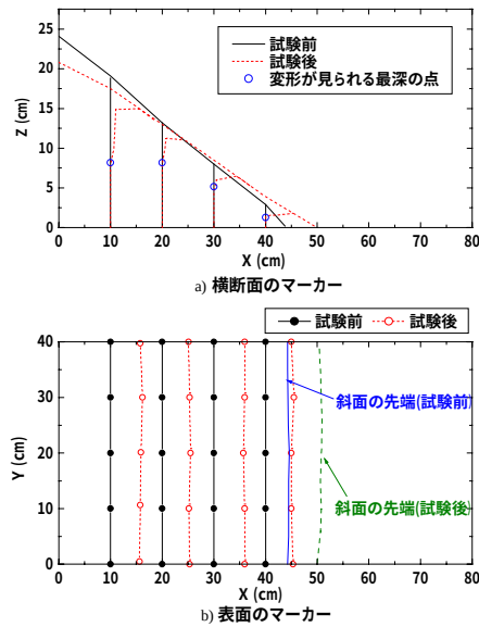
図-5 試験前後のマーカーの動き
