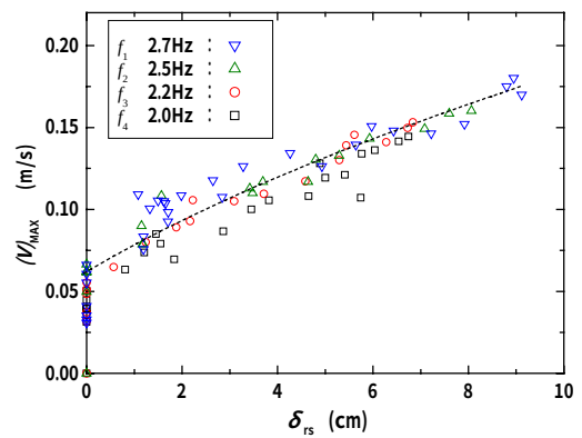
図-17 最大速度 (V)_{MAX} と水平方向の平均変位 \delta_{rs} の関係
