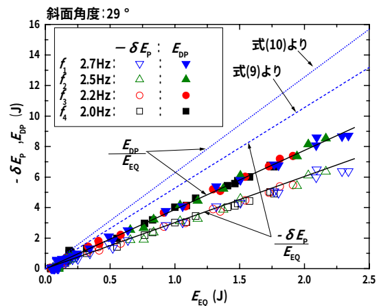
図-20 斜面角度 29^\circ の異なる振動数 f による振動エネルギー E_{EQ} と位置エネルギーの変化量 -\delta E_p 、消費エネルギー E_{DP} の関係
