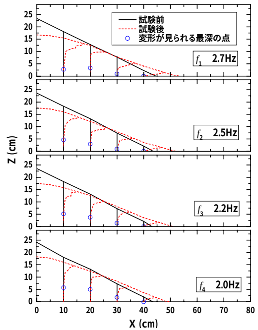
図-13 試験前後の横断面のマーカー
