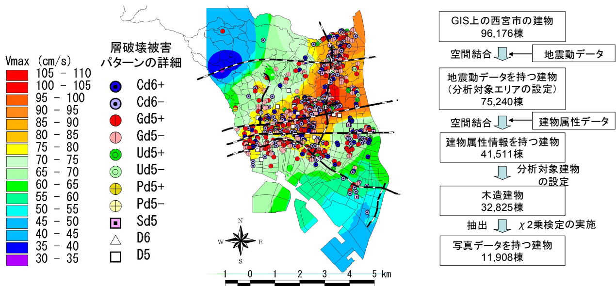
図-2 最大地表速度 (PGV) と層破壊建物の分布
