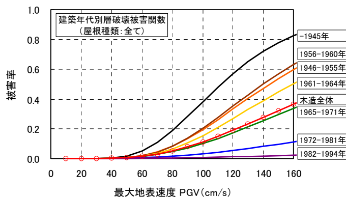
図-6 建築年代別層破壊被害関数
