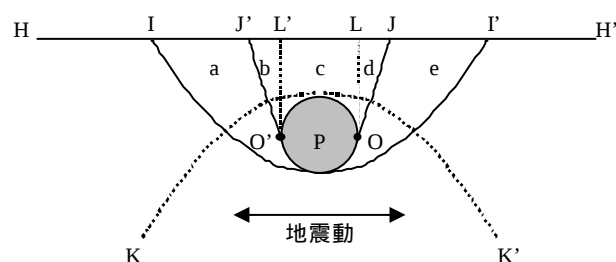
図-17 交番载荷を受ける埋設管
