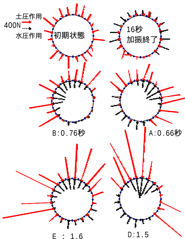
図-18 埋設管に作用する水圧と土圧
