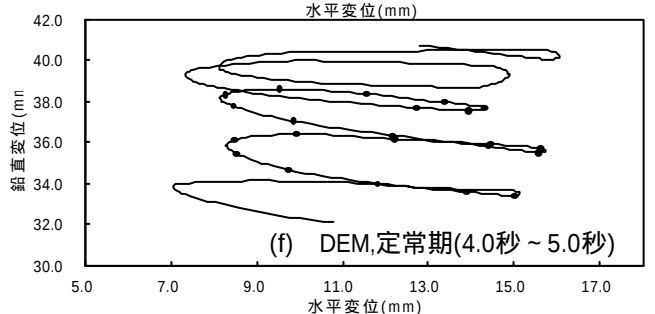
図-14 埋設管の描くオービット
