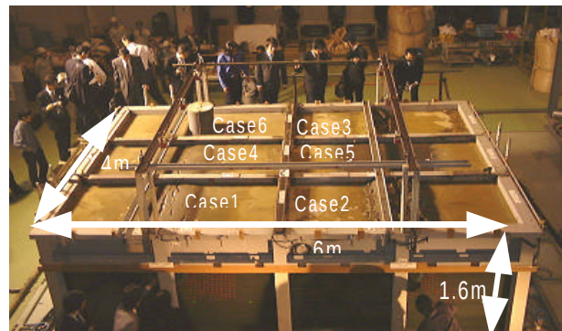
写真-1 加振終了後の土槽
