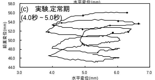
図-14 埋設管の描くオービット
