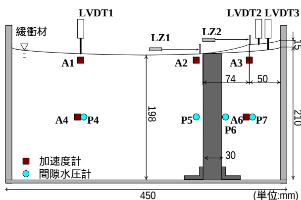
図-2 模型地盤概要 (Case2, 薬液改良 30mm)
