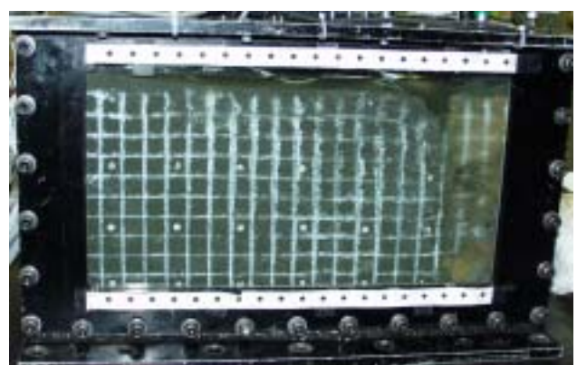
図-10 変形後の写真 (Case4, 薬液改良 70mm)
