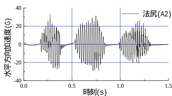
図-20 法尻での水平方向加速度 (Case4)
