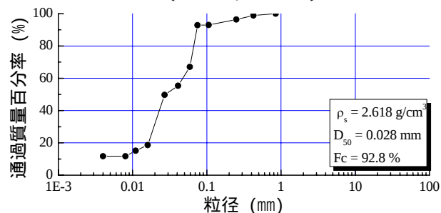
図-6 シルト砂の粒径加積曲線
