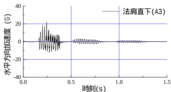
図-16 法尻直下での水平方向加速度 (Case1)
