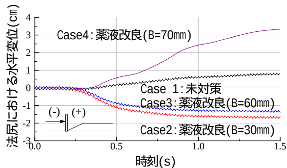
図-13 法尻における水平変位
