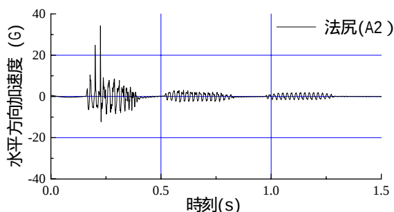
図-15 法尻での水平方向加速度 (Case1)
