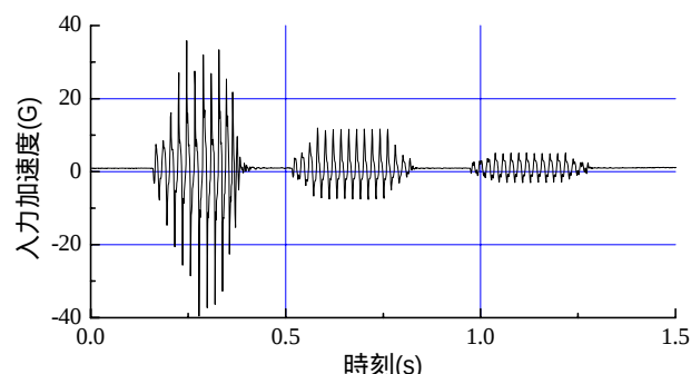
図-5 入力加速度 (Case1, 未対策)
