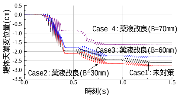
図-12 堤体天端の変位量
