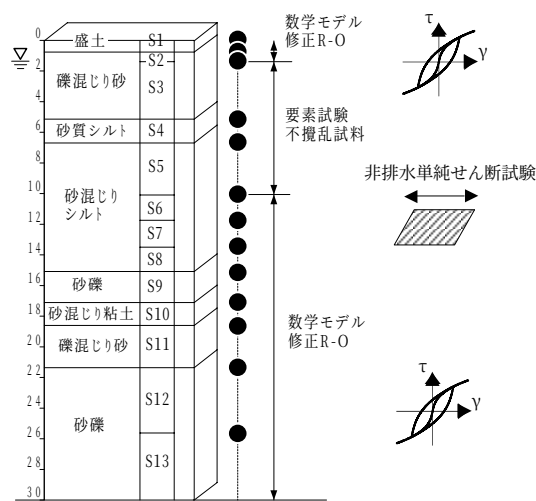
図-8 実験対象断面図
