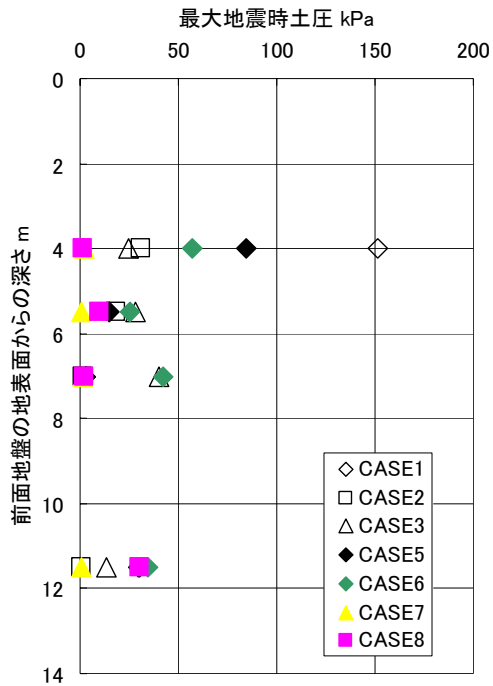
図-7 前面側杭の地震時主働土圧 (Step2)
