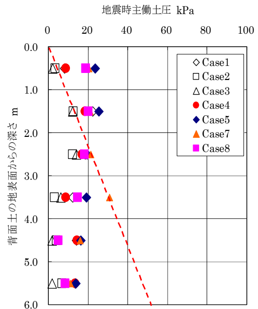
図-3 地震時主働土圧（Step1）
