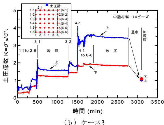
図-7 土圧係数の経時変化（締固め開始～加振前）
