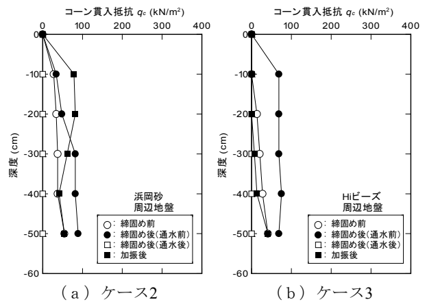
図-4 コーン貫入抵抗深度分布（周辺地盤）
