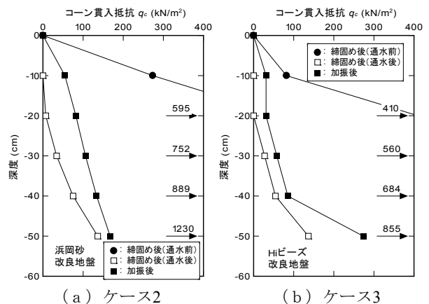
図-5 コーン貫入抵抗深度分布（改良地盤）
