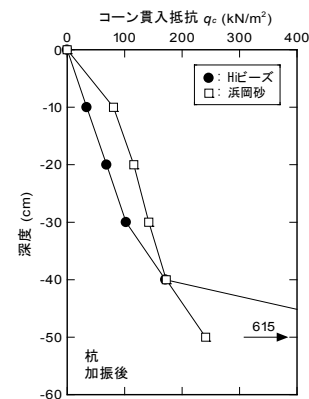
図-6 コーン貫入抵抗深度分布（杭）
