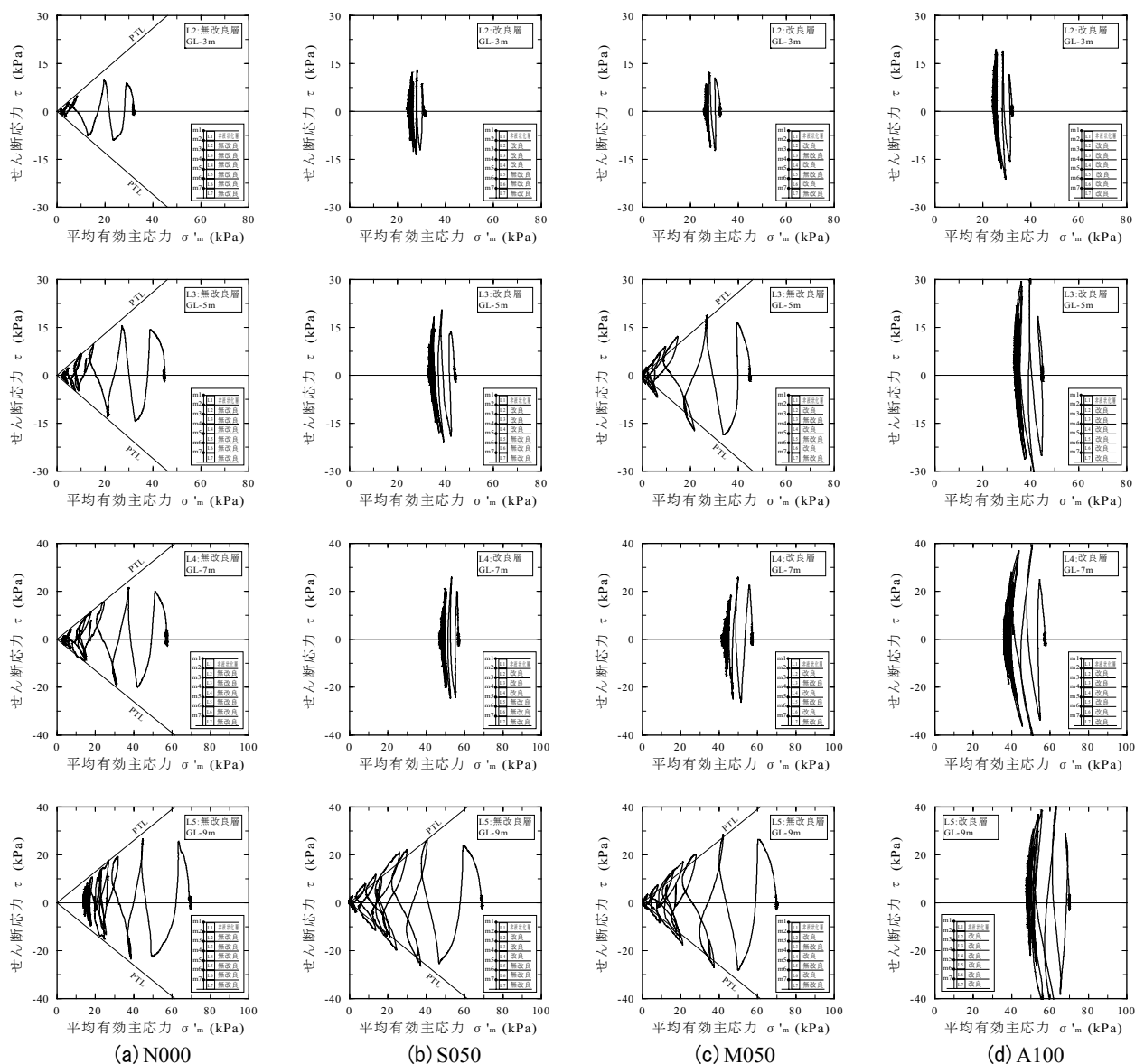
図-5 有効応力経路
