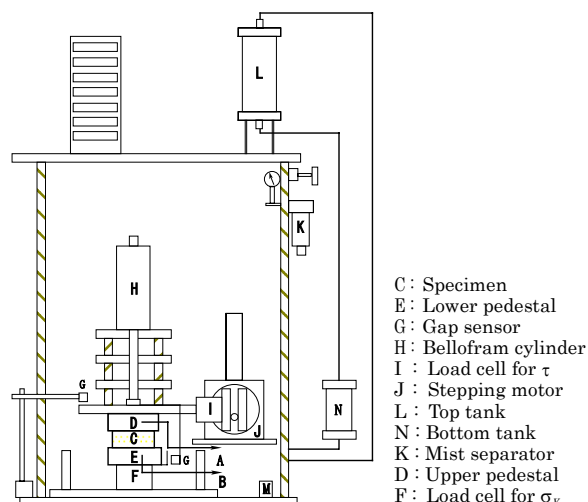
図-1 簡易単純せん断試験装置
