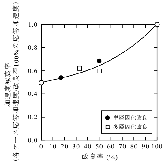
図-11 加速度減衰率と改良率の関係
