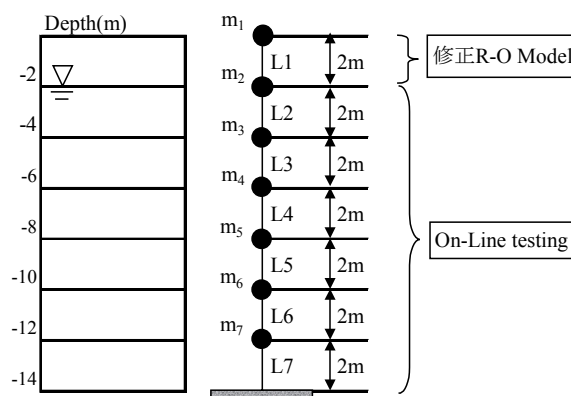
図-2 地盤モデル
