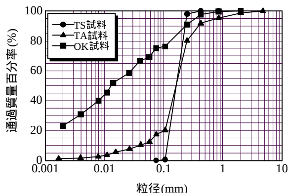
図-3 使用した試料の粒度加積曲線
