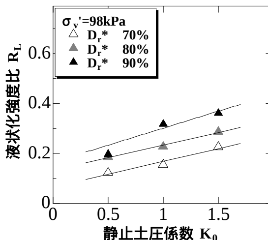
図-6(b) R_L と静止土圧係数の関係 (TA 試料)
