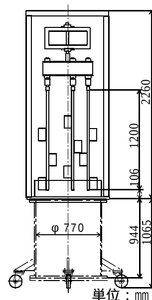
図-4 地盤再利用攪拌装置
