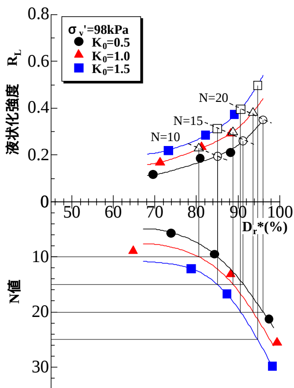
図-7(b) N 値と静止土圧係数の関係 (TA 試料)
