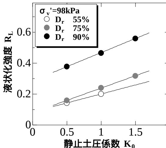
図-6(a) R_L と静止土圧係数の関係 (TS 試料)
