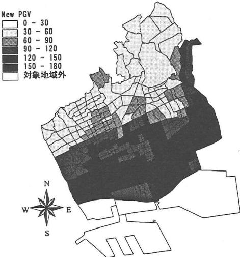
図-3 灘区の推定地震動 10)
