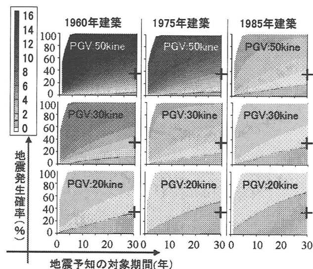
図-6 予知対象期間と地震発生確率の影響
