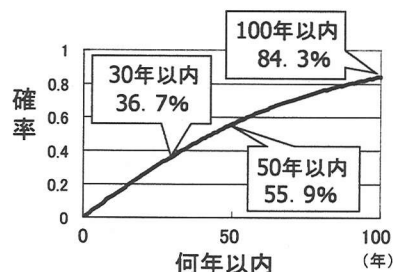
図-3 東海地震の発生確率
