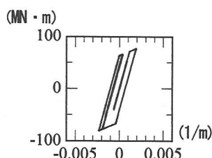
図-12 タワー基部 M- \phi 関係 (免震デバイス使用)
