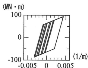
図-11 タワー基部 M- \phi 関係 (基本タワー)
