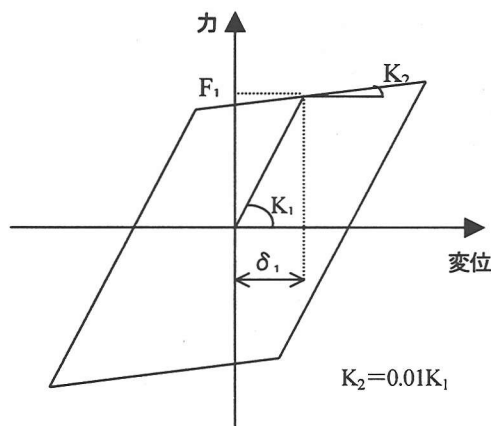
図-3 免震デバイスの履歴
