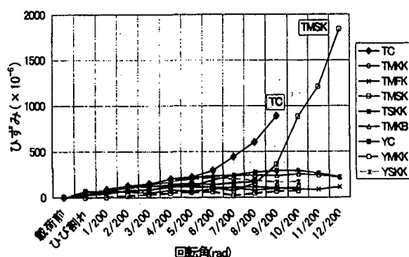
図一 6 圧縮側帯鉄筋の歪み一回転角曲線
