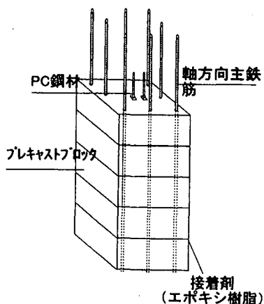
図-1 PRC橋脚の概念
