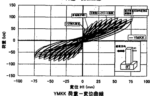
図-4 Tシリーズ、Yシリーズの荷重変位曲線の代表例
