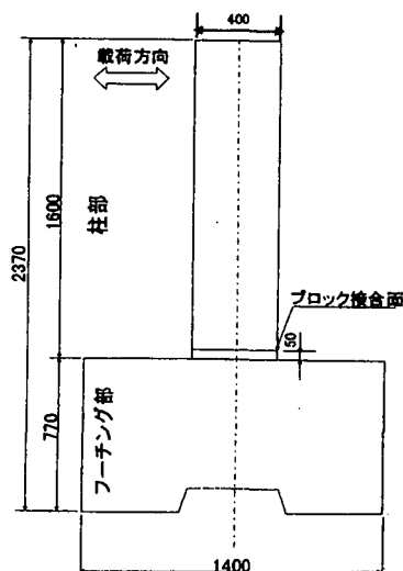
図-2 供試体の基本寸法
