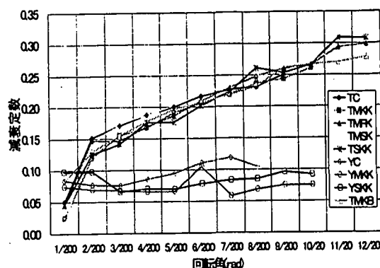
図一 7 橋脚の回転角と減衰定数の関係
