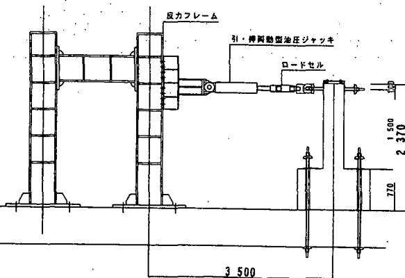
図-3 水平載荷試験装置
