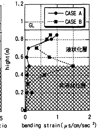
図-7 最大曲げひずみ分布 (隅杭)
