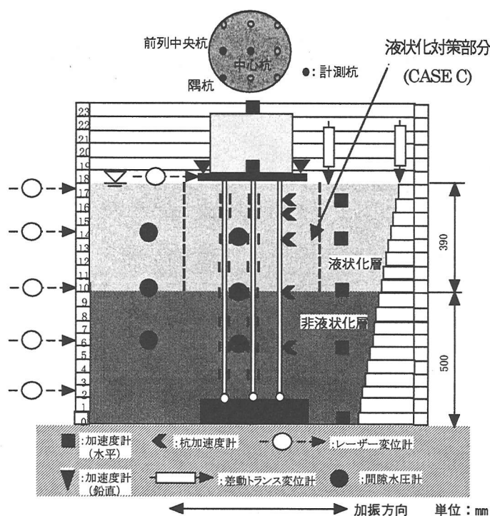
図一 実験システム
