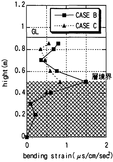
図－9 最大曲げひずみ分布 (隅杭)
