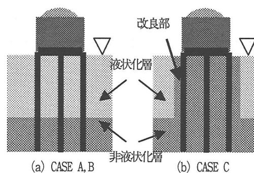
図二 実験模式図
