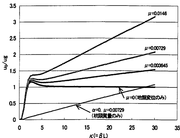
図-2 杭体変位と \kappa の関係 (杭頭回転フリー)
