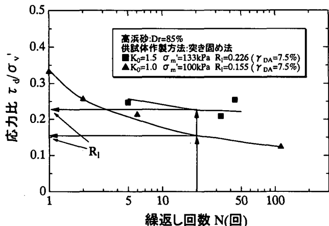
図-6 繰返しねじりせん断試験における 応力比～液状化回数関係
