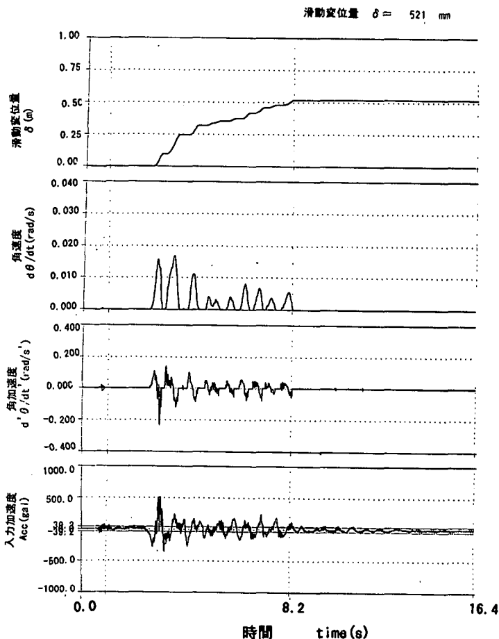
図-7 ニューマーク法による滑動解析結果
