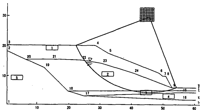
図-6 フェレニウス法による安定計算
