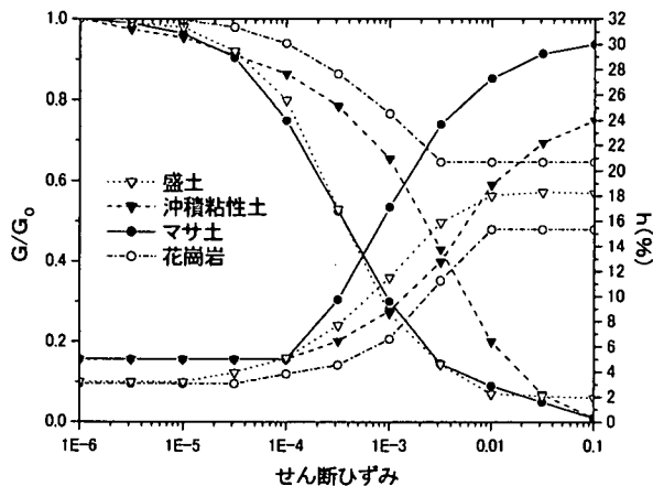
図－４ 動的物性値のひずみ依存性の関係
