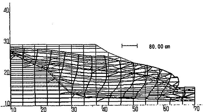
(d) 動的解析による変形図
