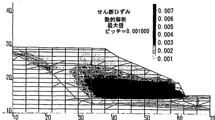
(c) 動的せん断ひずみ分布図
