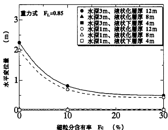
図 13. 細粒分含有率と水平変位量の関係 (重力式)
