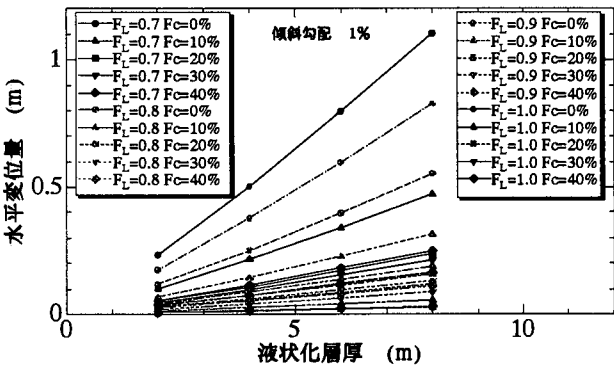
図7. 液状化層厚と水平変位量の関係 (勾配1%)
