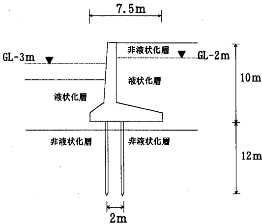
図6. 重力式護岸モデル
