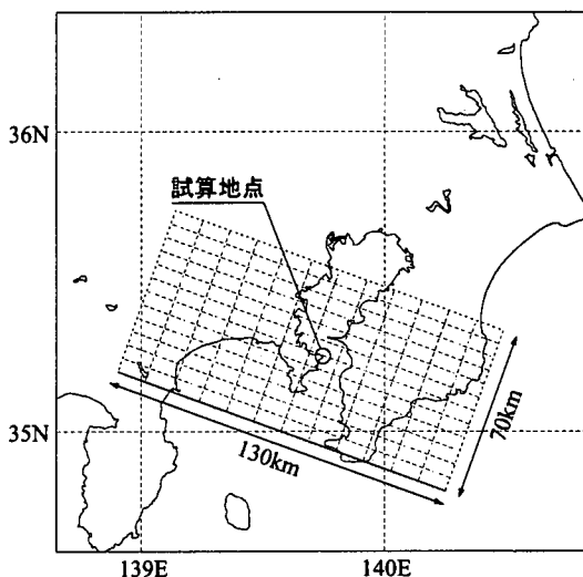
図-1 試算に用いた1923年関東地震の断層モデル
