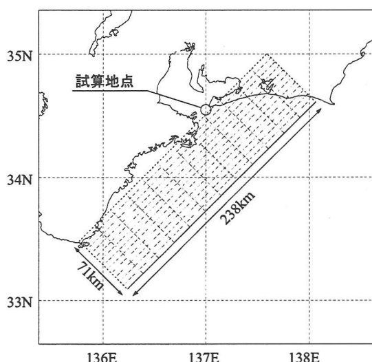
図-5 試算に用いた1944年南海地震の断層モデル
