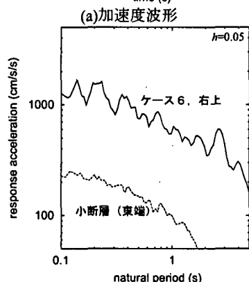
図-7 試算した加速度波形とその応答スペクトルの例
