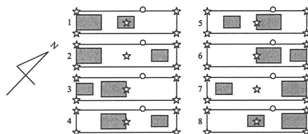
図-6 設定した断層モデルの震源及びアスぺリティの位置(☆:震源、○:試算地点)
