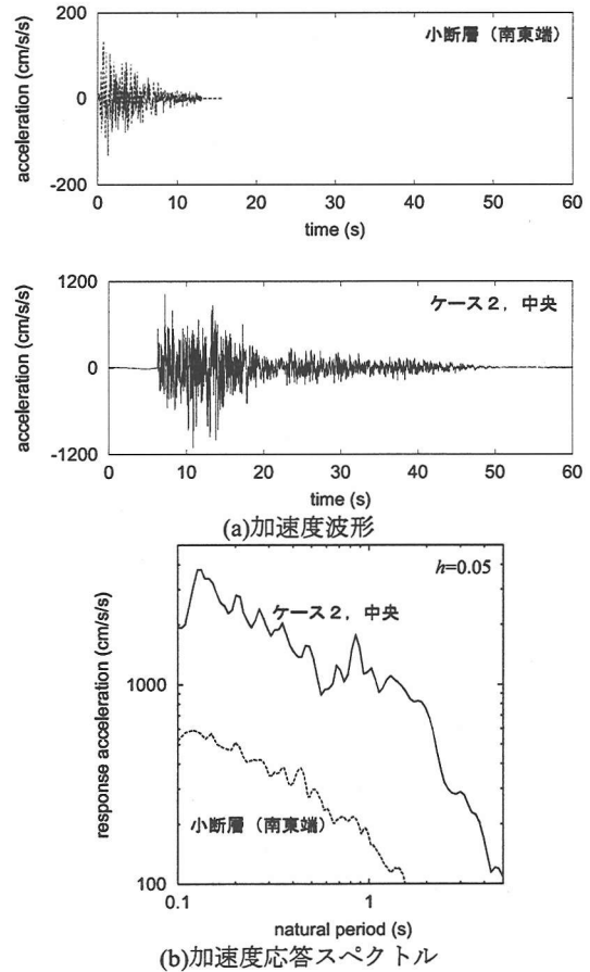
図-3 試算した加速度波形とその応答スペクトルの例
