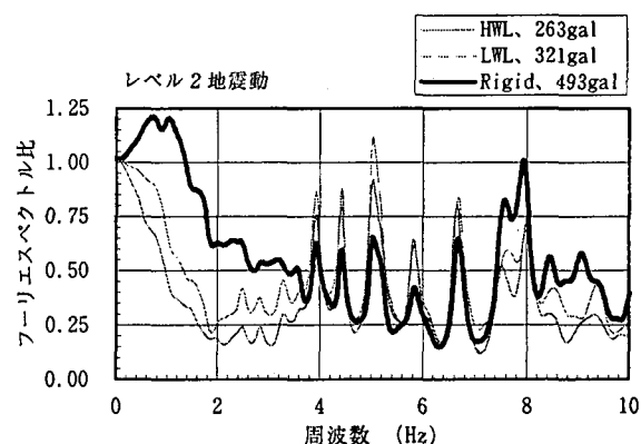
図 5-2 #2 函体の加速度フーリエスペクトル比
