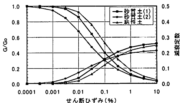
図 3-3 G/G_0 \sim \gamma , h \sim \gamma 曲線
