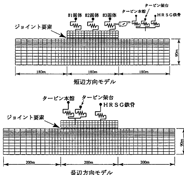
図 3-1 解析モデル
