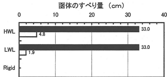
図 5-4 函体の滑り量の比較
