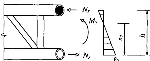
図-3 アーチリブ断面の力学状態
