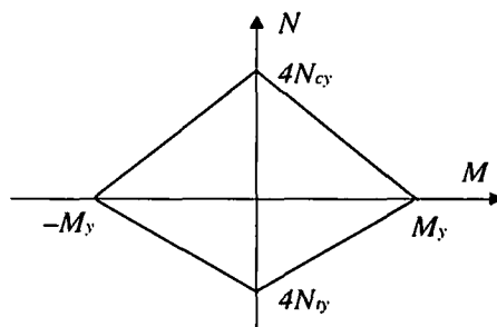
図-4 曲げモーメントと軸力の相関関係
