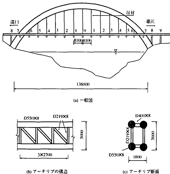
図-1 対象橋の構造 (単位: mm)
