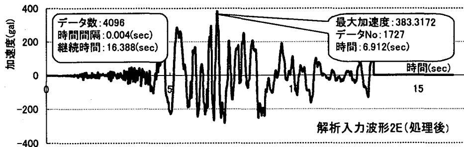
図-4 入力波形
