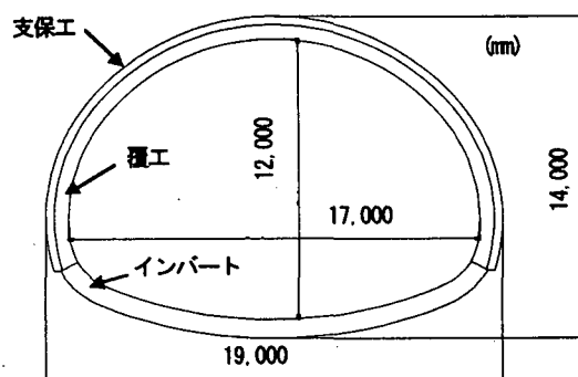
図-1 トンネル横断面の概略
