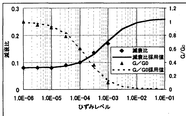
図-3 G- \gamma 、h- \gamma 曲線
