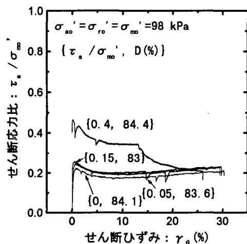
(b) 初期せん断応力の影響
