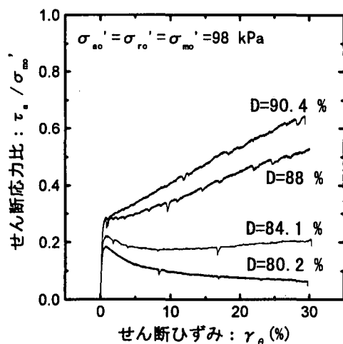
(a) 締固め密度の影響
