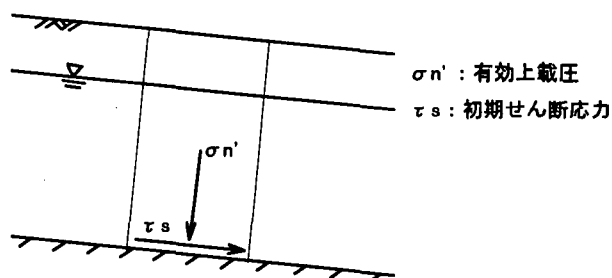
図9 単純斜面
