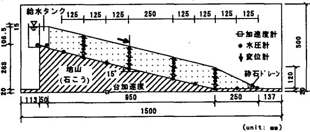
図 1 実験模型
