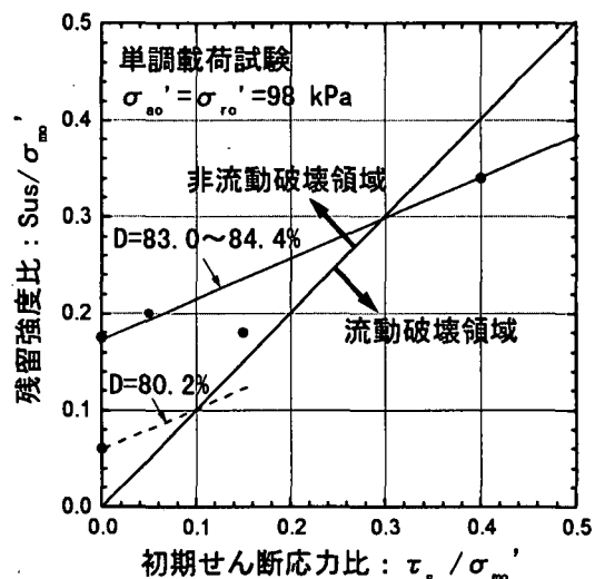
図8 残留強度と初期せん断応力の関係
