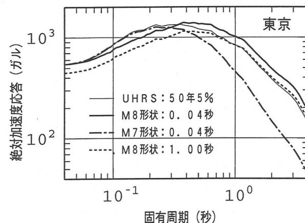
図-4 一般ハザード応答スペクトルと各周期の地震分布に基づくスペクトル形状の比較
