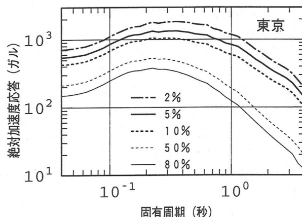
図-2 減衰5%の一般ハザード応答スペクトルの例。数字は50年間の超過確率
