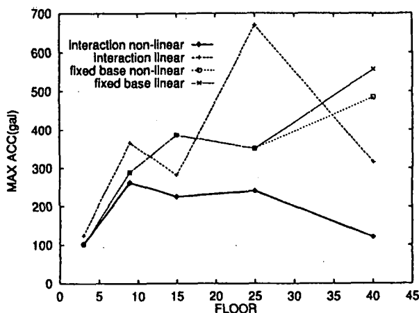
図-6 Roma-C 地点での、4種類の解析モデルによる、5種類のビルの最上階の最大応答加速度 (NS成分) の比較。
