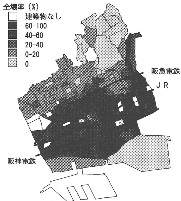
図-6 町丁目ごとの木造の全壊率
