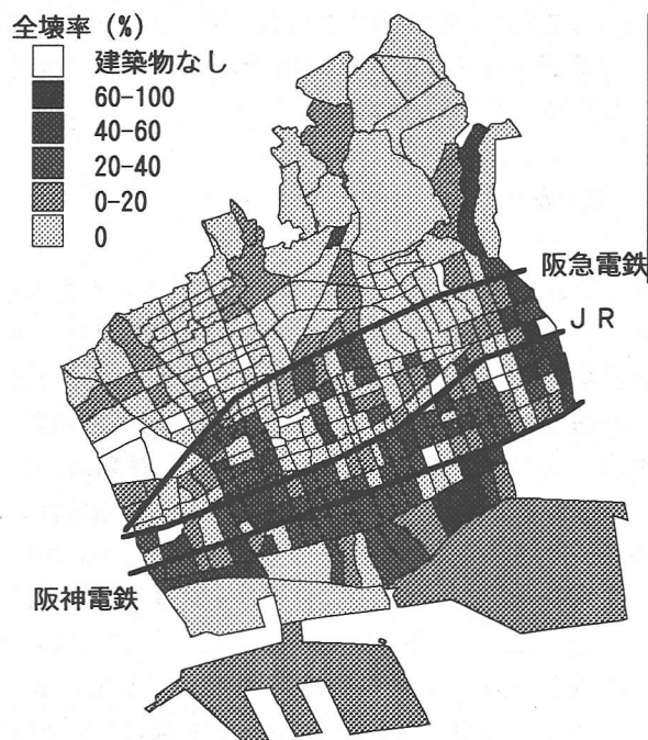
図-8 町丁目ごとのRC造の全壊率
