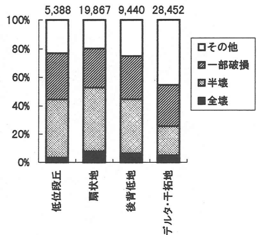
図-7 地盤分類別の木造建物（2階以上・重い屋根）被害率
