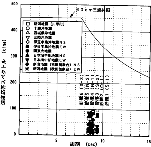
図-3 貯槽の一次固有周期と速度応答スペクトル
